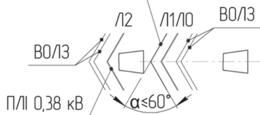
Схема встановлення опори ПЛ 0,38 кВ
