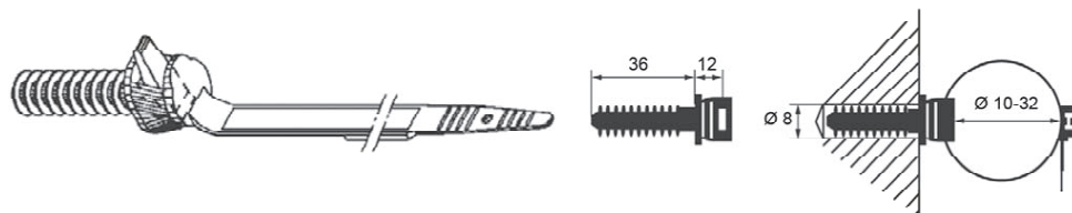
Фасадний кронштейн СН8 С32 (Позиція 56)
