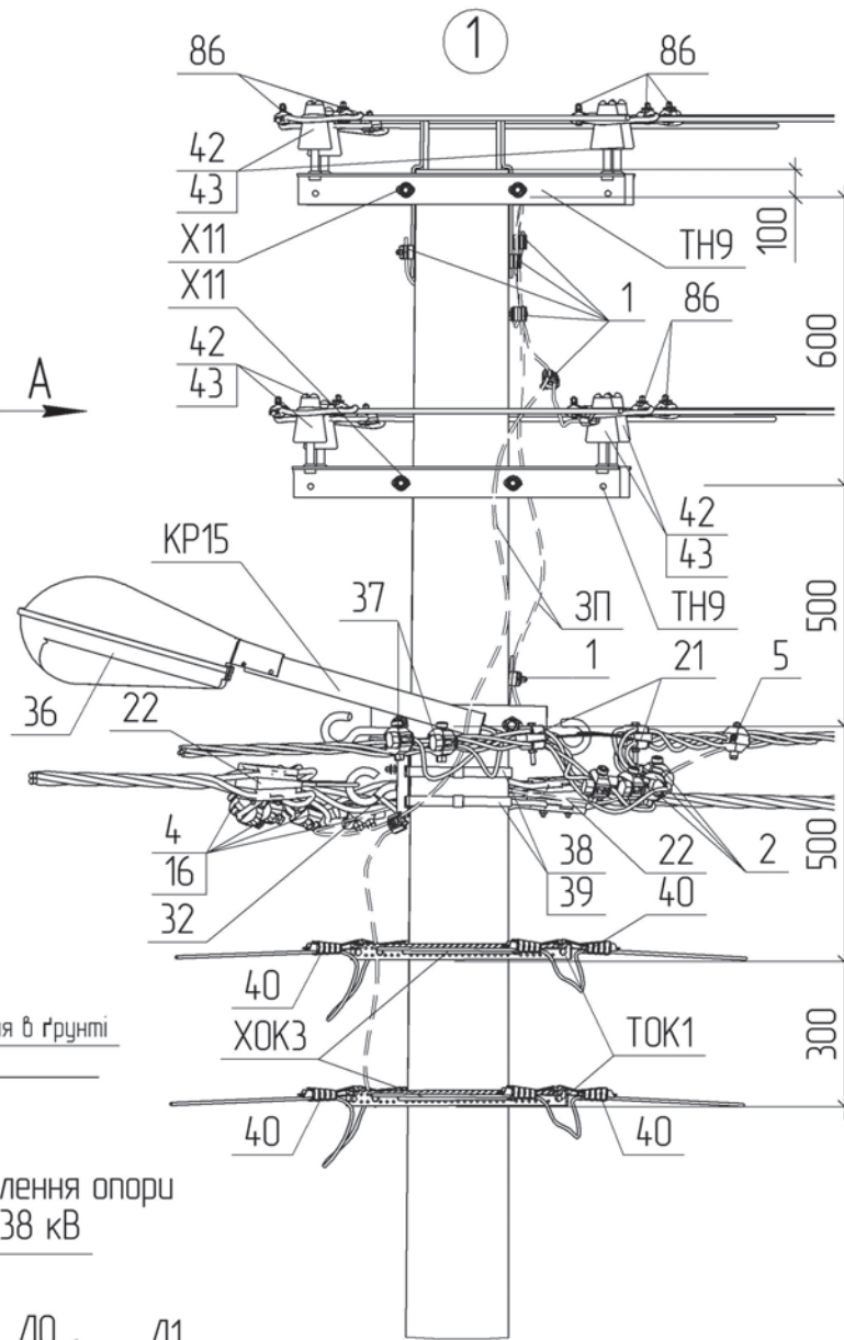
Магістраль П/Лі 0,38 кВ
