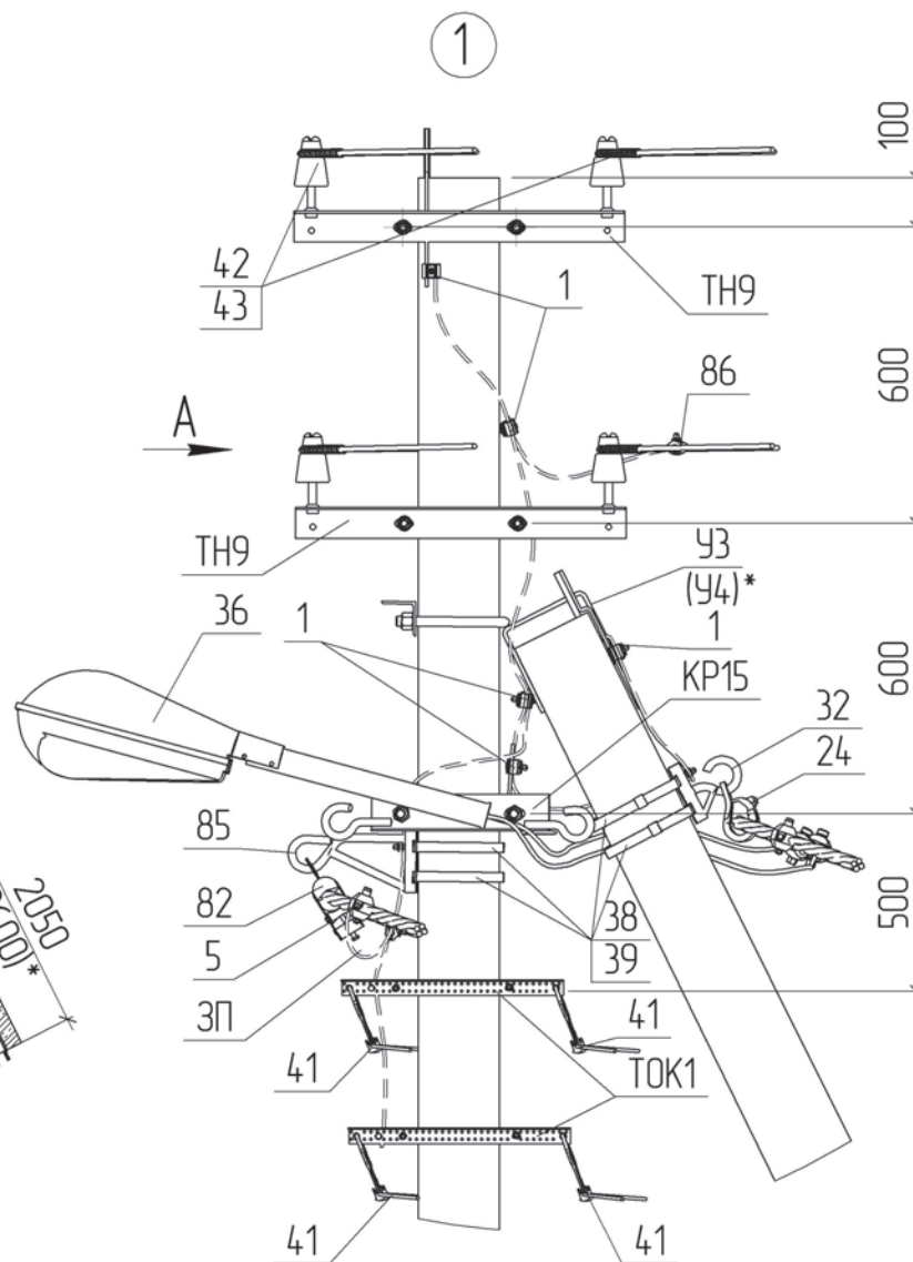
Схема встановлення опори ПЛ 0,38 кВ
