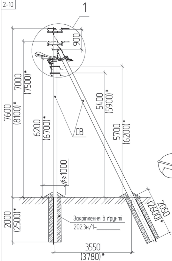
Схема встановлення опори ПЛ 0,38 кВ
