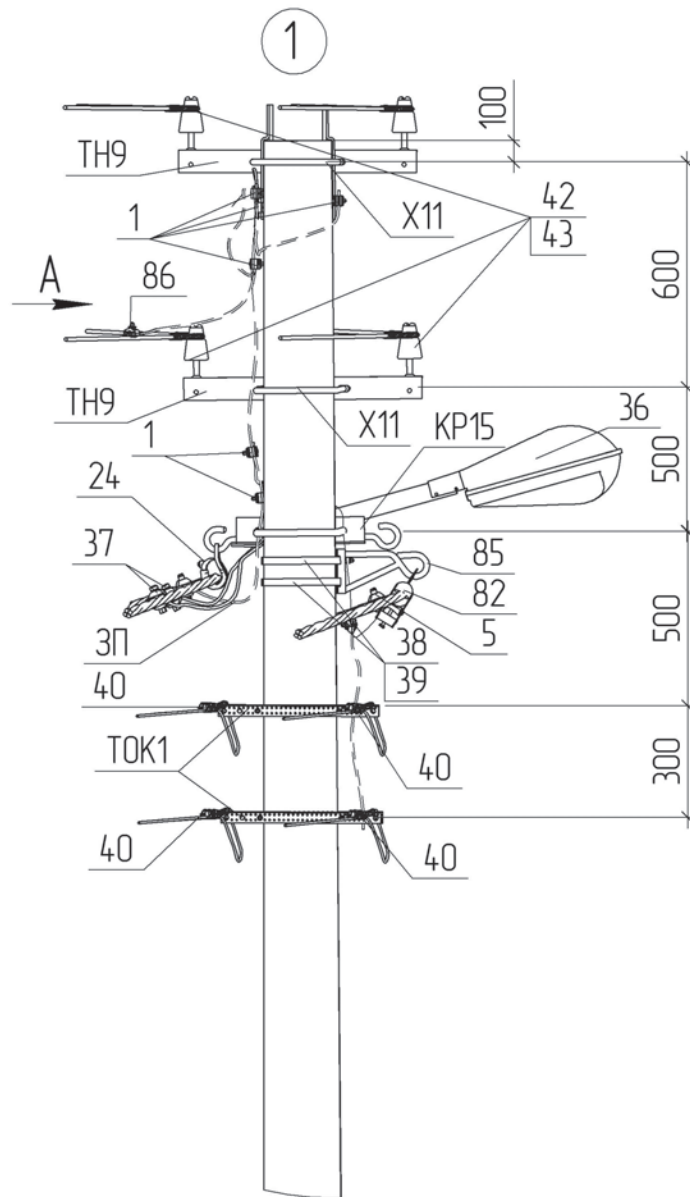
Схема встановлення опори Магістраль П/Л 0,38 кВ
