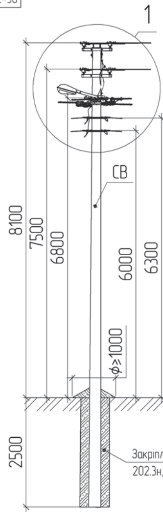
Схема встановлення опори Магістраль П/Лі 0,38 кВ
