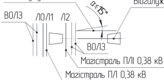
Схема встановлення опори
