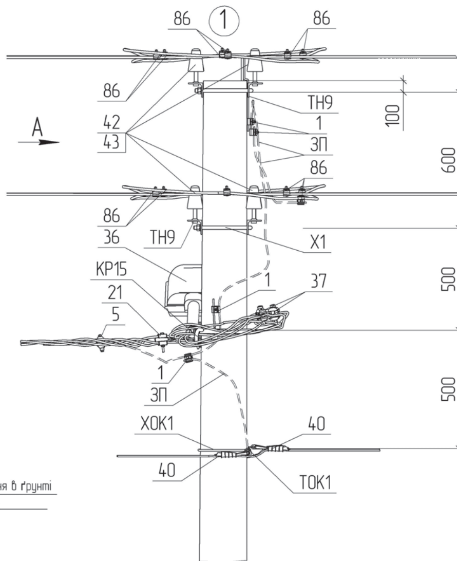
Схема встановлення опори
