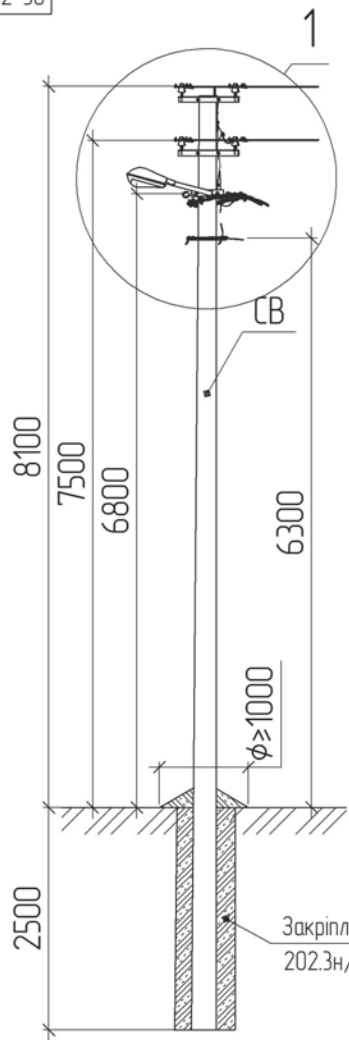
Схема встановлення опори Магістраль П/Л 0,38 кВ ( T_{max}=0,5кН )
