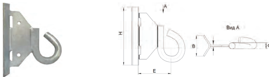
Гак бандажний GHSO 12 (Позиція 49)
