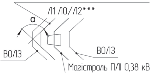
Схема встановлення опори Магістраль П/Л 0,38 кВ ( T_{max}=0,5кН )
