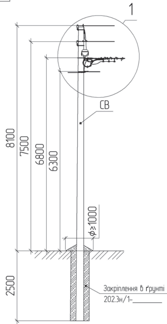
Схема встановлення опори
