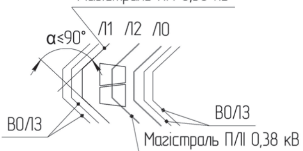
Схема встановлення опори Магістраль ПЛ 0,38 кВ
