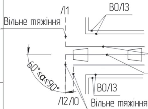
Схема встановлення опори
