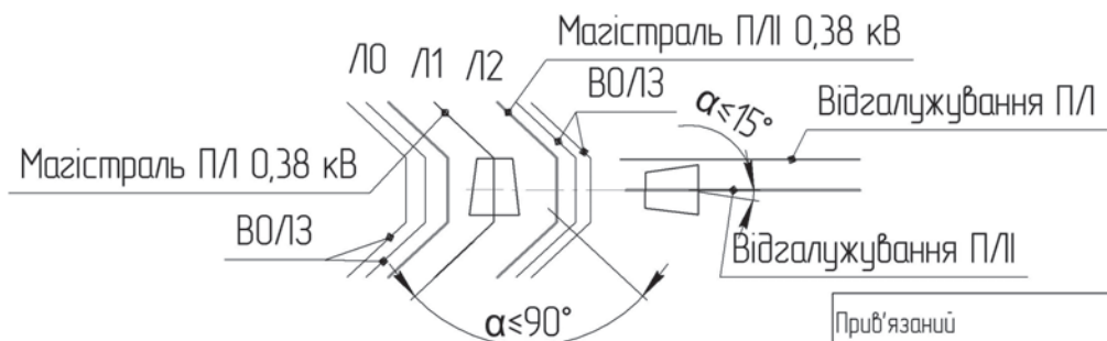
Схема встановлення опори
