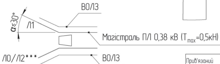
Схема встановлення опори
